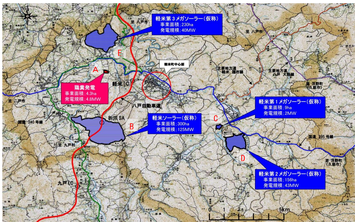
図 再生可能エネルギー発電の整備を促進する区域の位置
