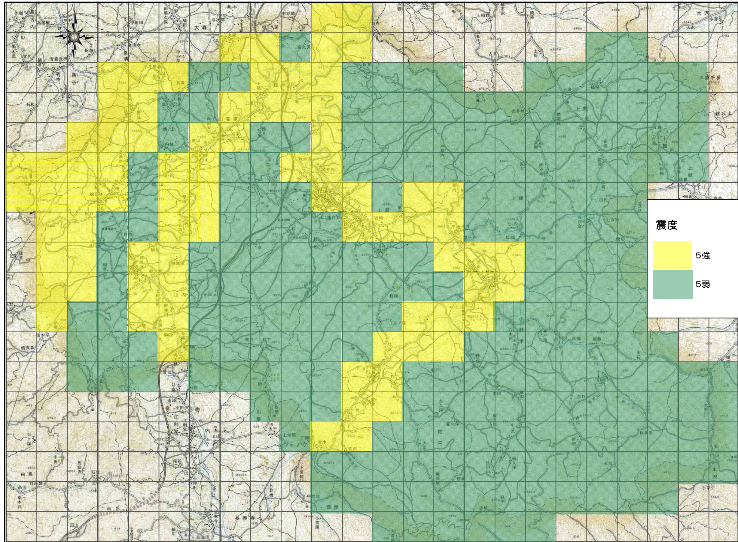
図 震度の予想結果図(想定:三陸沖北部の地震)
